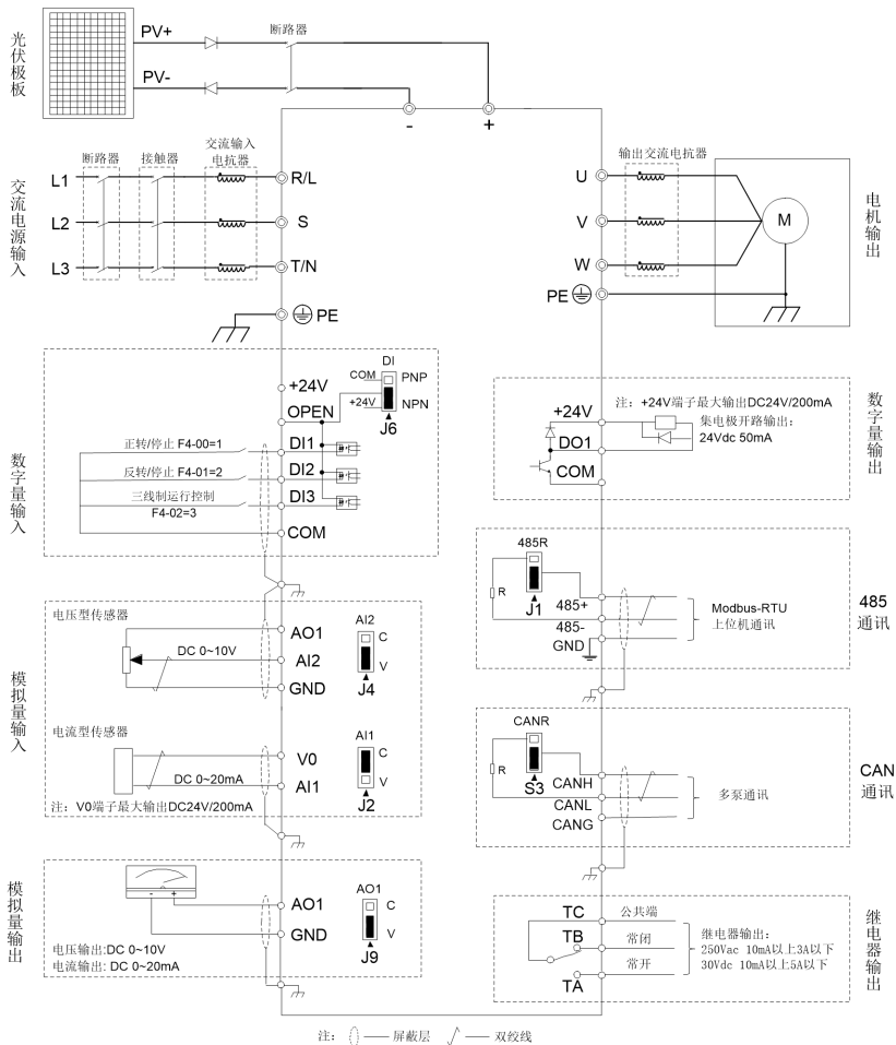
图 3.2-1 变频器标准接线示意图
