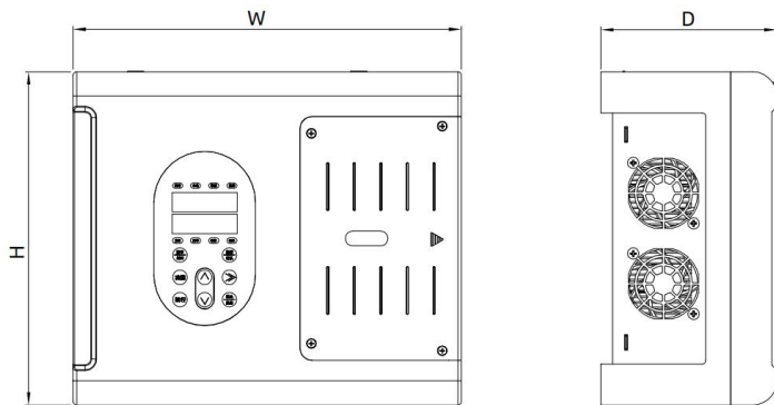
图 2.5-1 产品外形及安装尺寸示意图
