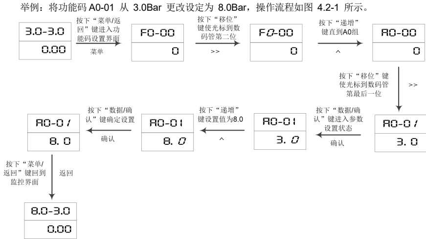
图 4.2- 1 LED 键盘操作流程图
