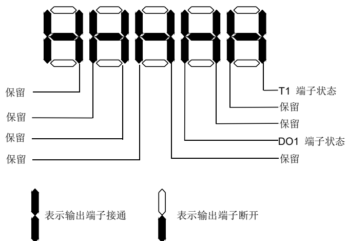
图 5.4-2 输出端子接通/断开状态示意图
