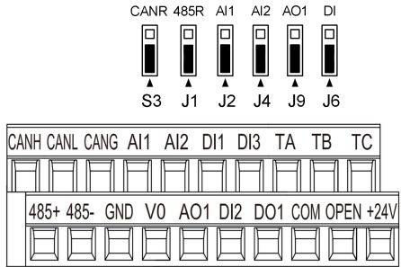
图 3.3-1 控制回路端子示意图
