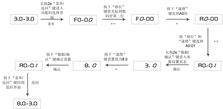
图 4.2- 1 LED 键盘操作流程图
