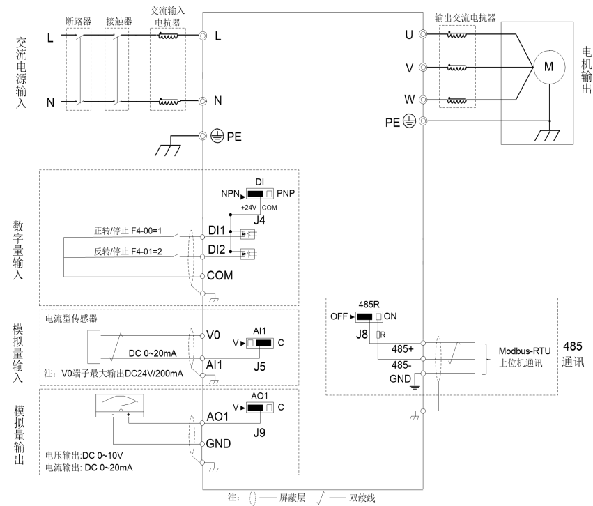
图 3.2-1 变频器标准接线示意图
