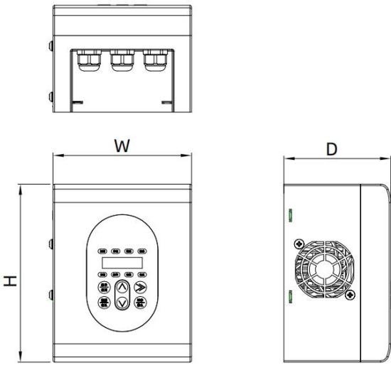
图 2.5-1 产品外形及安装尺寸示意图
