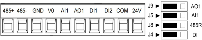
图 3.4-1 控制回路端子示意图
