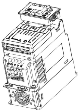
图 3.3-1 操作面板的拆卸和安装示意图
