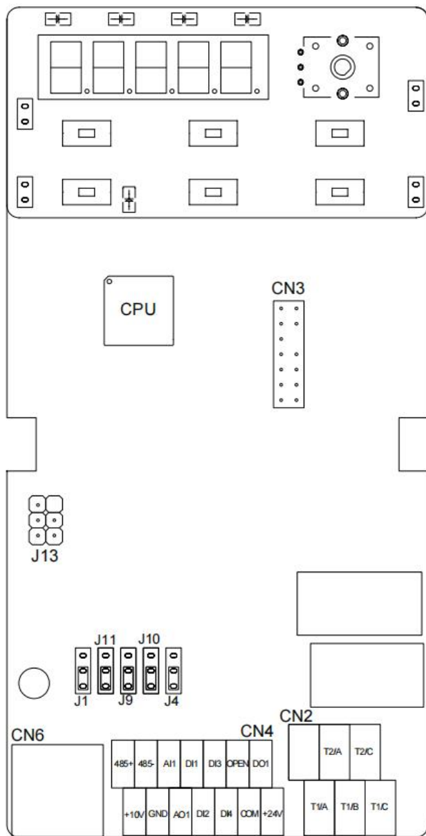
图 3.5-2 7.5kW~22kW 控制板布局示意图
