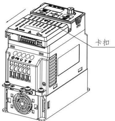
图 3.3-2 5.5kW 以下塑胶外壳盖板的拆卸和安装示意图
