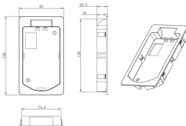
图 2.5-1 外引键盘外形尺寸
