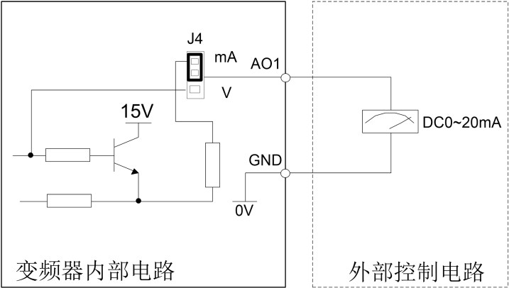
图. 3.5-9 模拟量输出端子输出电流信号接线示意图
