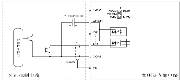
图 3.5-5 NPN 模式使用外部电源
