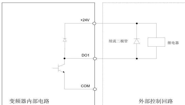
图. 3.5-7 使用集电极开路输出的数字输出端子
