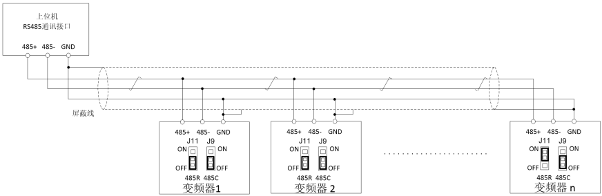
图. 3.5-12 单台/多台变频器 RS485 通讯端子接线图
