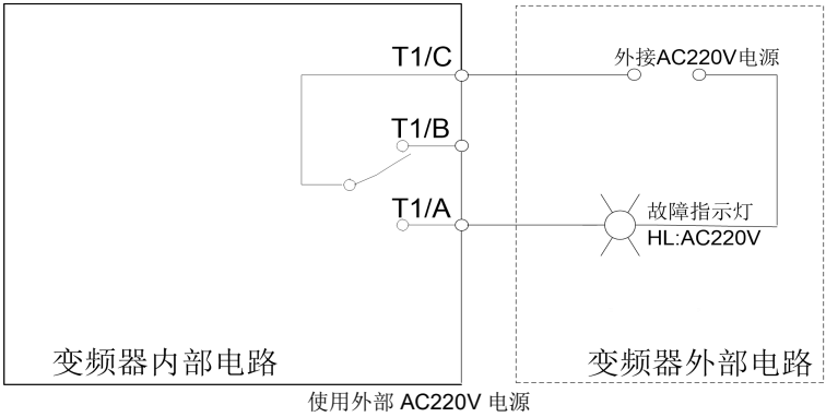
图. 3.5-10 继电器输出端子接线示意图
