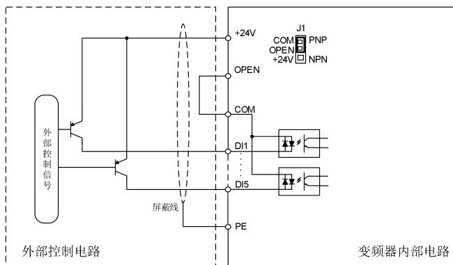
图 3.5-4 PNP 模式使用内部电源
