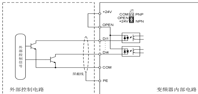
图 3.5-3 NPN 模式使用内部电源
