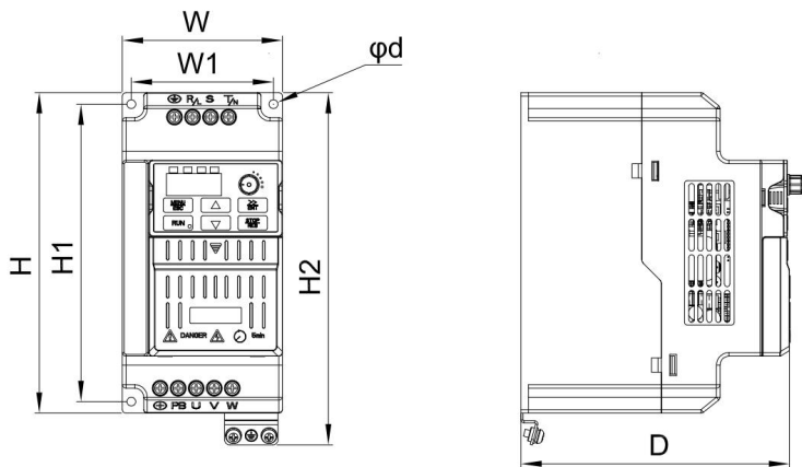
图 2.4-2 (三相 380V: 4.0kW-5.5kW ; 单相、三相 220V: 2.2kW )
