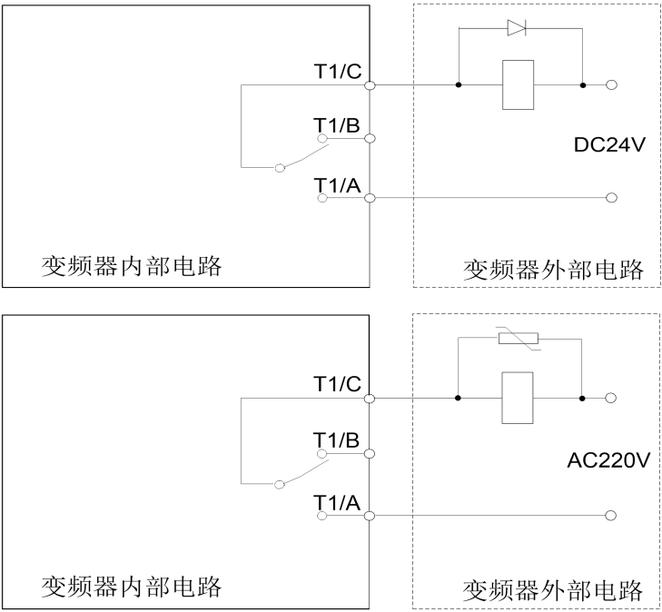
图. 3.5-11 继电器输出端子抗干扰处理
