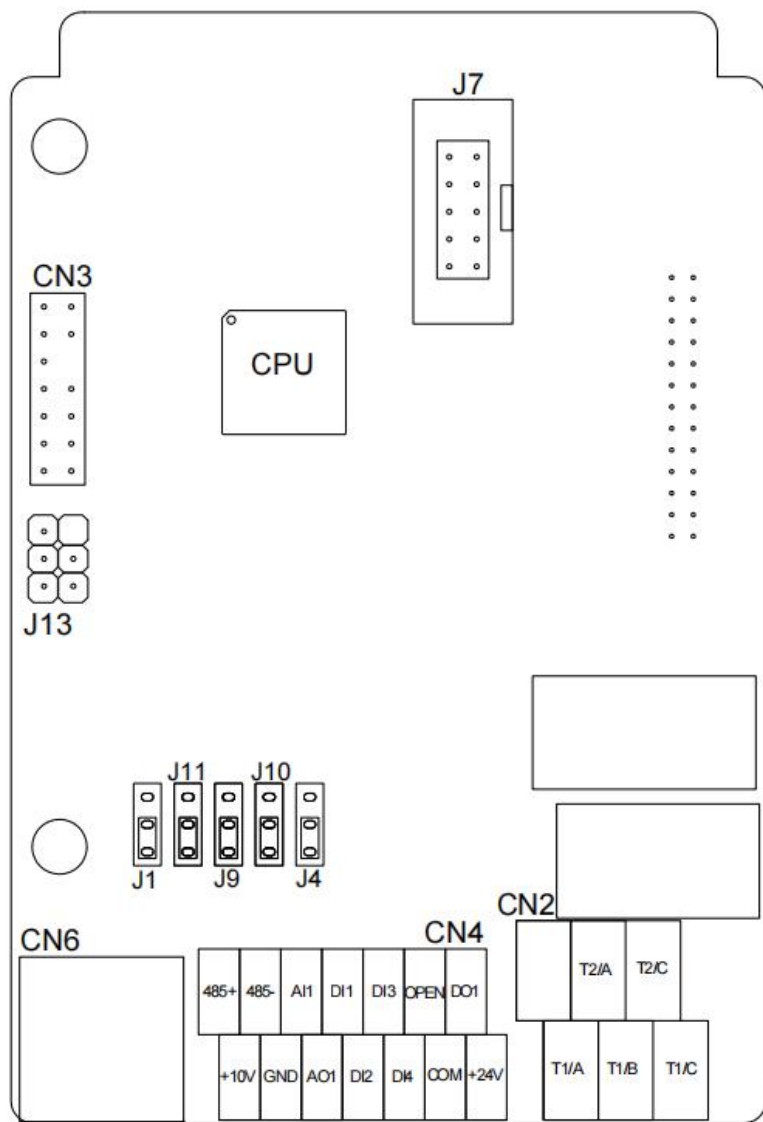
图 3.5-1 0.4kW~5.5kW 控制板布局示意图
