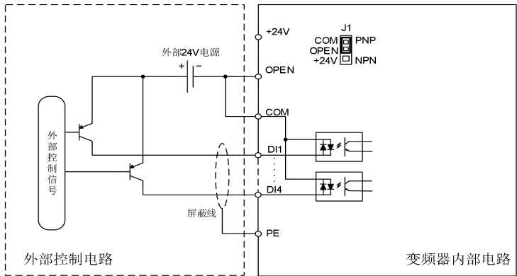
图 3.5-6 PNP 模式使用外部电源
