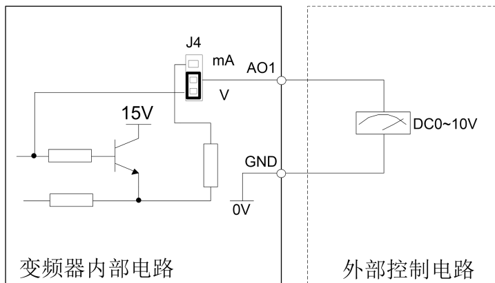
图 3.5-8 模拟量输出端子输出电压信号接线示意图
