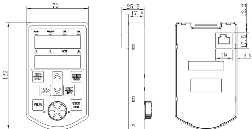
图 2.5-1 外引键盘外形尺寸
