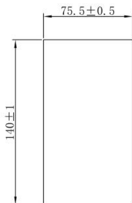
图 2.5-3 外引键盘托盘安装开孔尺寸
