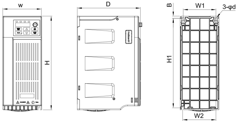
图 2.4-3 适应机型（三相 380V：7.5kW-11kW、15kW-22kW）
